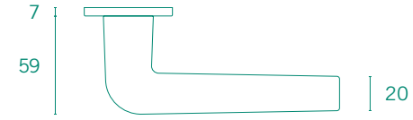
APRILE FUNKIA rozeta R SLIM 7mm
