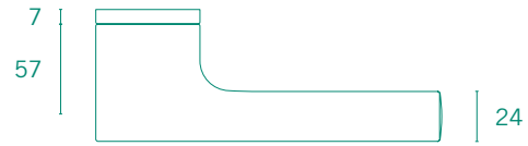
APRILE LUPINA rozeta RTH SLIM 7mm
