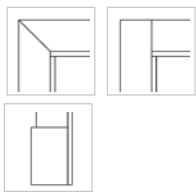
7. Ościeżnica regulowana z cokołem dolnym Listwa opaskowa 80/20
