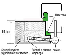
PROFIL SKRZYDŁA
