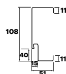
Rysunek techniczny
