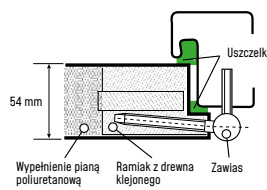
PROFIL SKRZYDŁA
