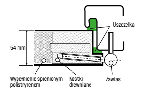
PROFIL SKRZYDŁA
