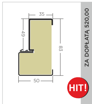
ościeżnica Termo ODS68
