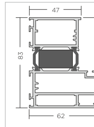
ościeżnica Termo ALU 68
