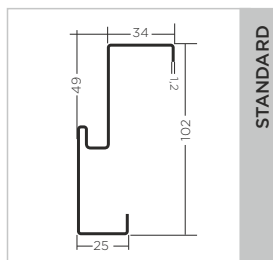
ościeżnica PU68
