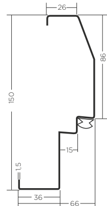
OŚCIEŻNICA PM84/150
