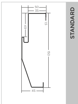
ościeżnica stalowa PD68/150
