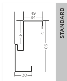
ościeżnica PU56
